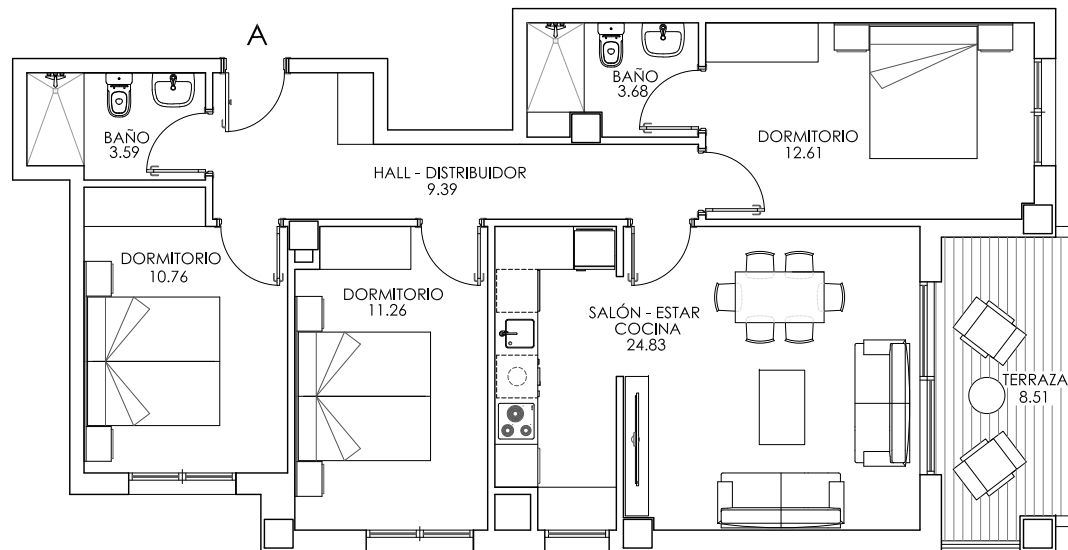
PLANTA TIPO DE VIVIENDAS
